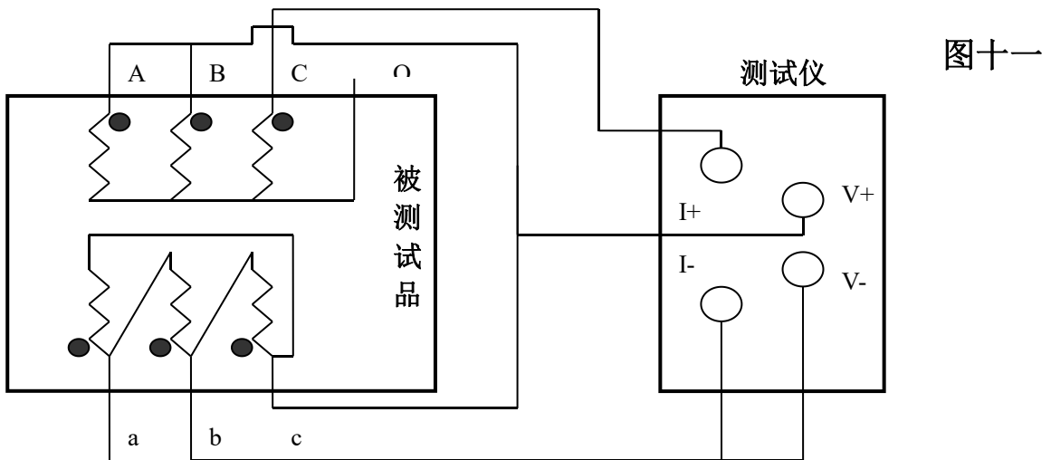
图九、十、十一分别为测量低压 R_{ac} 、 R_{ba} 、 R_{bc} 的接线方法
